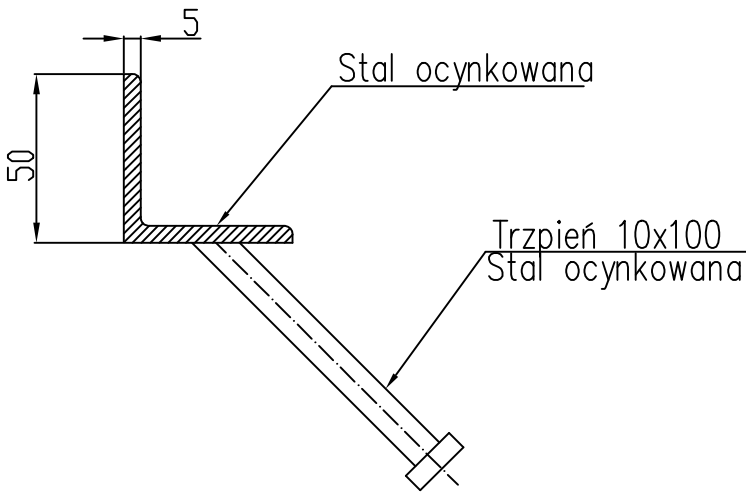
Rzut z góry Skala 1:2
