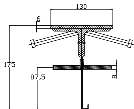
CONECTO SINUS 06NCE130-5D-T8 h=175 Przekrój
