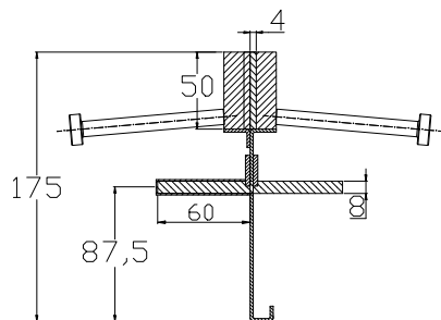
CONECTO SINUS 04NS50-4D-T8 h=175 Przekrój
