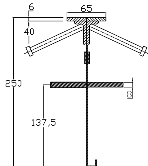
CONECTO SINUS 06NCC65/40x20-5D-T8 h=250 Przekrój
