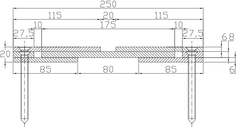
CONECTO ZIGZAG 06NZ250/20-R S80K20 Przekrój
