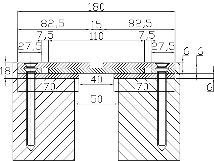
Conecto Sinus 06NC180/18-R S50K15 PRZEKRÓJ
