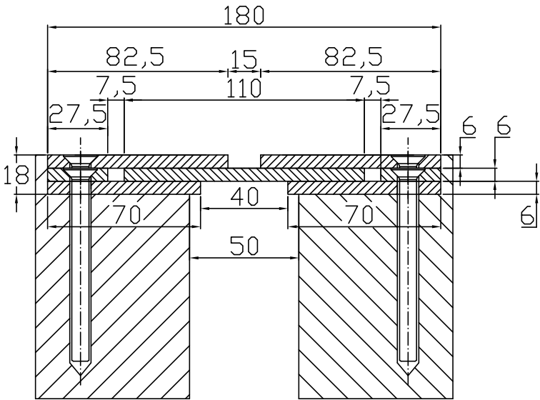
Conecto Sinus 06NC180/18-R S50K15 PRZEKRÓJ
