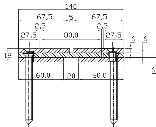
Conecto Sinus 06NC140/18-R S20K5 Przekrój
