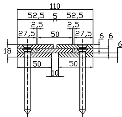
Conecto Sinus 06NC110/18-R S10K5 Przekrój
