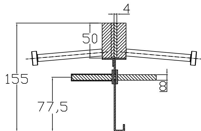
CONECTO SINUS 04NS50-4D-T8 h=155 Przekrój
