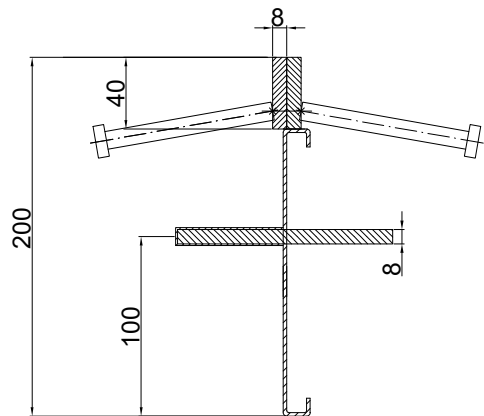
CONECTO DOWEL 08NA40-5D-T8 h=200 Przekrój
