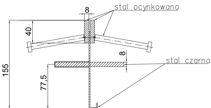
Conecto Dowel 08NA40-5D-T8 h=155 Przekrój
