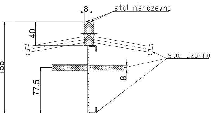
Conecto Dowel 08NA40-5D-T8 h=155 Przekrój
