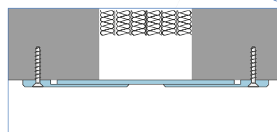
sufitowa wersja nakładkowa
