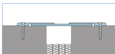
podłogowa wersja nakładkowa
