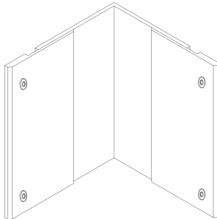
PROFIL DYLATACJNY WA 210 CV RZUT AKSONOMETRYCZNY
