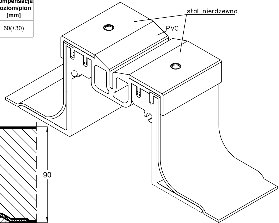
PROFIL DYLATACJNY GA 63.30.90 L RZUT AKSONOMETRYCZNY
