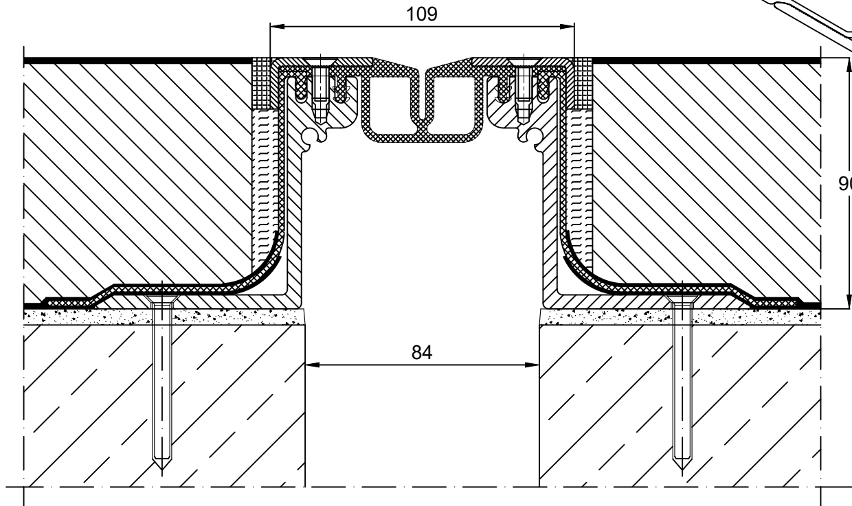
PROFIL DYLATACJNY GA 63.30.90 L PRZEKRÓJ
