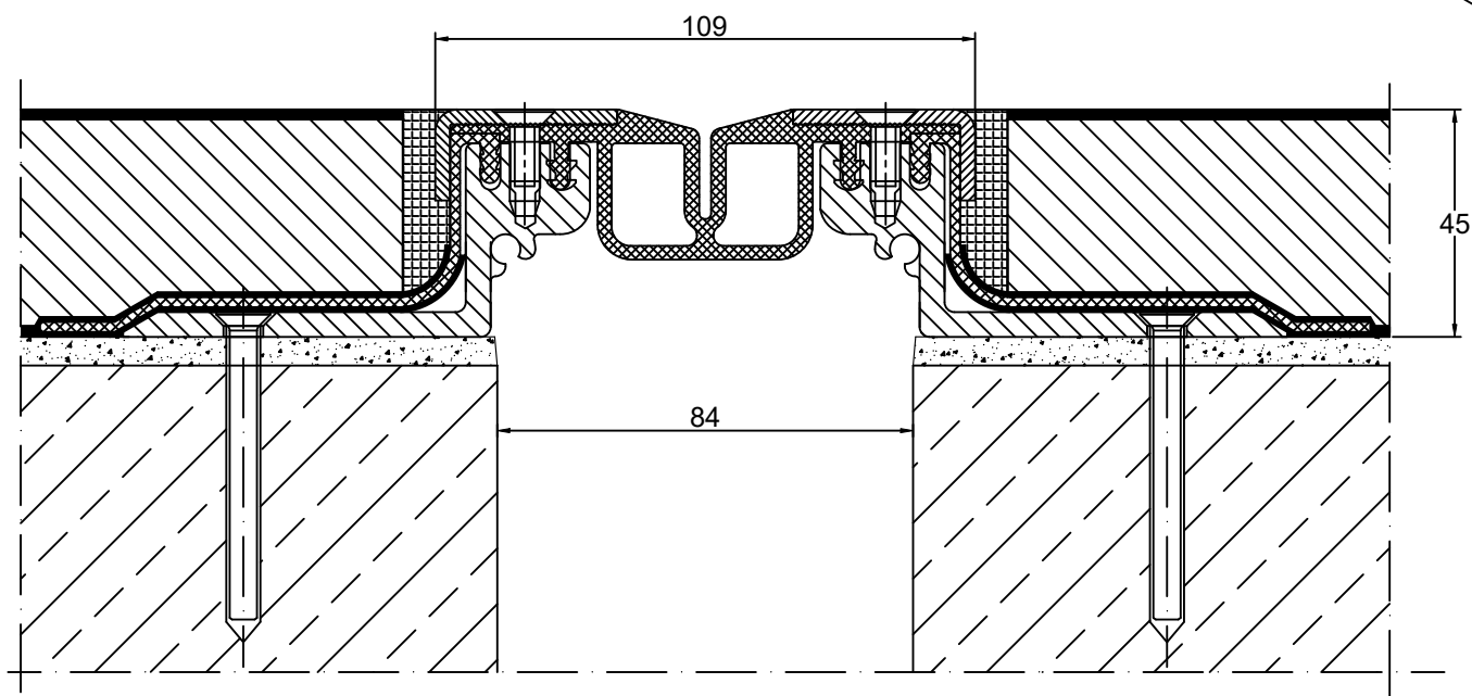
PROFIL DYLATACJNY GA 63.30.45 S PRZEKRÓJ
