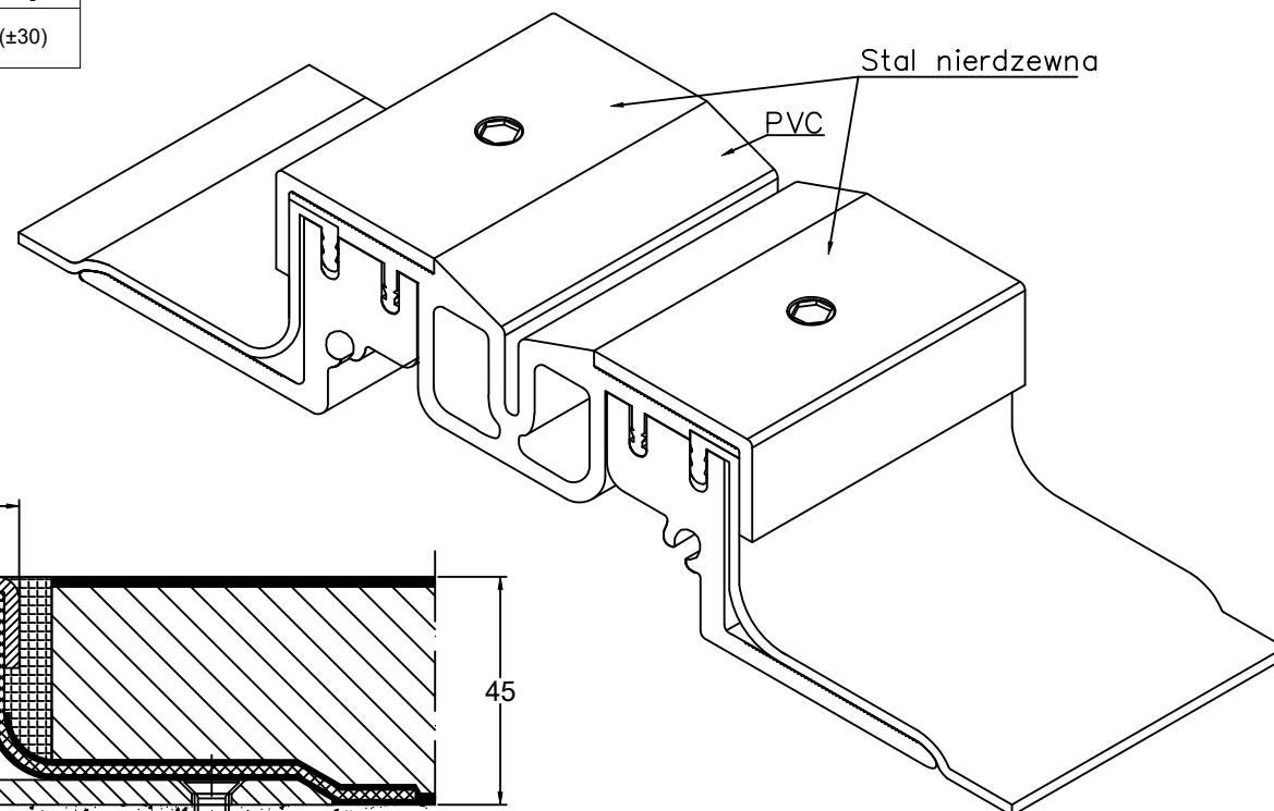
PROFIL DYLATACJNY GA 63.30.45 S PRZEKRÓJ
