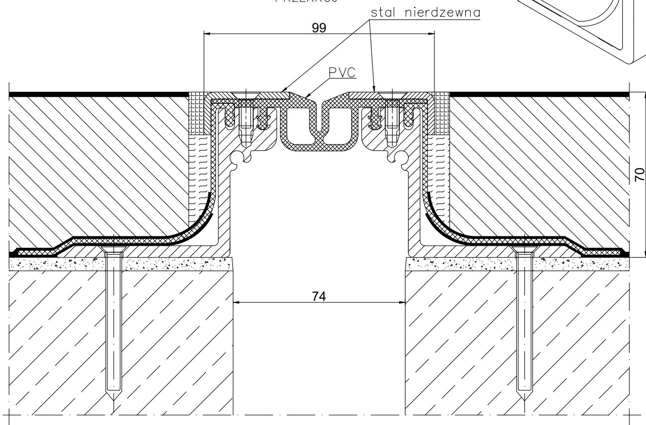
CONECTO GA 50.20.70 L PRZEKRÓJ
