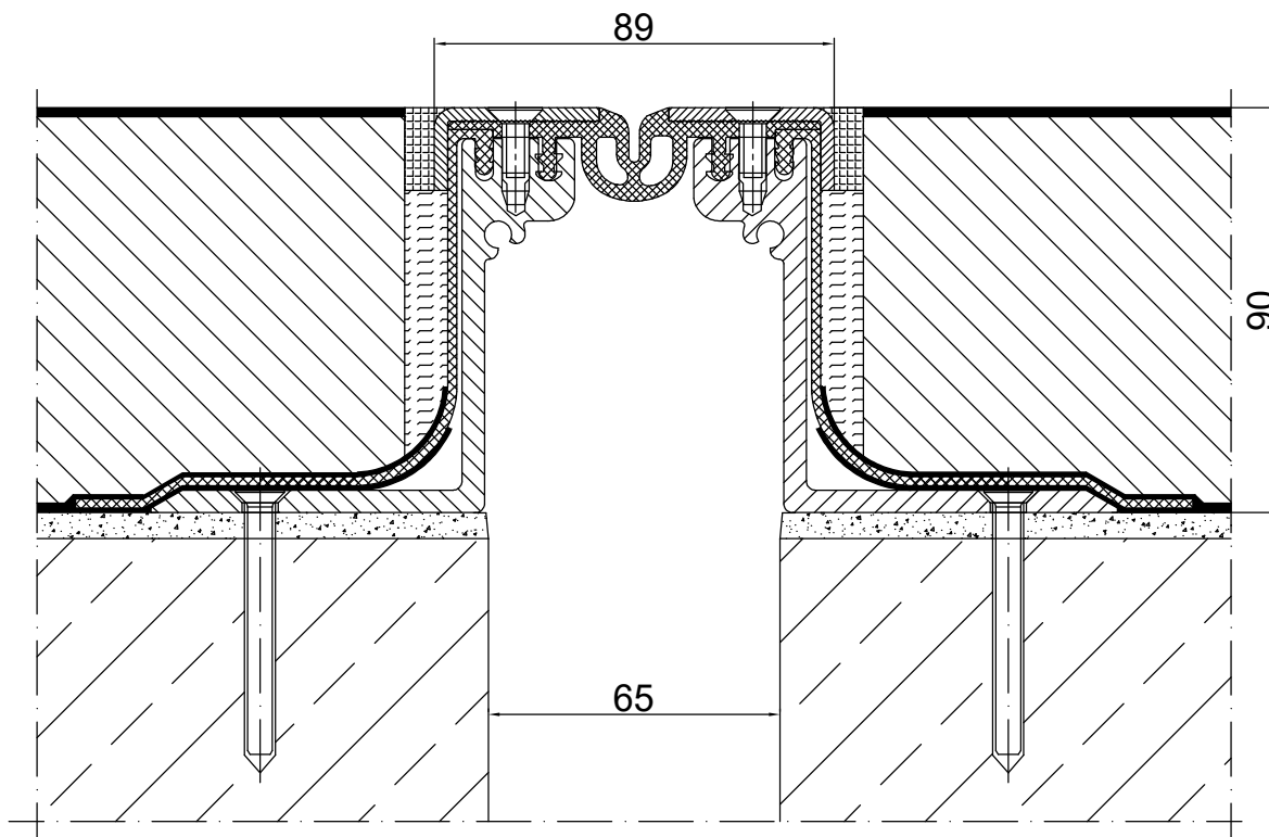
CONECTO GA 43.10.90 L PRZEKRÓJ
