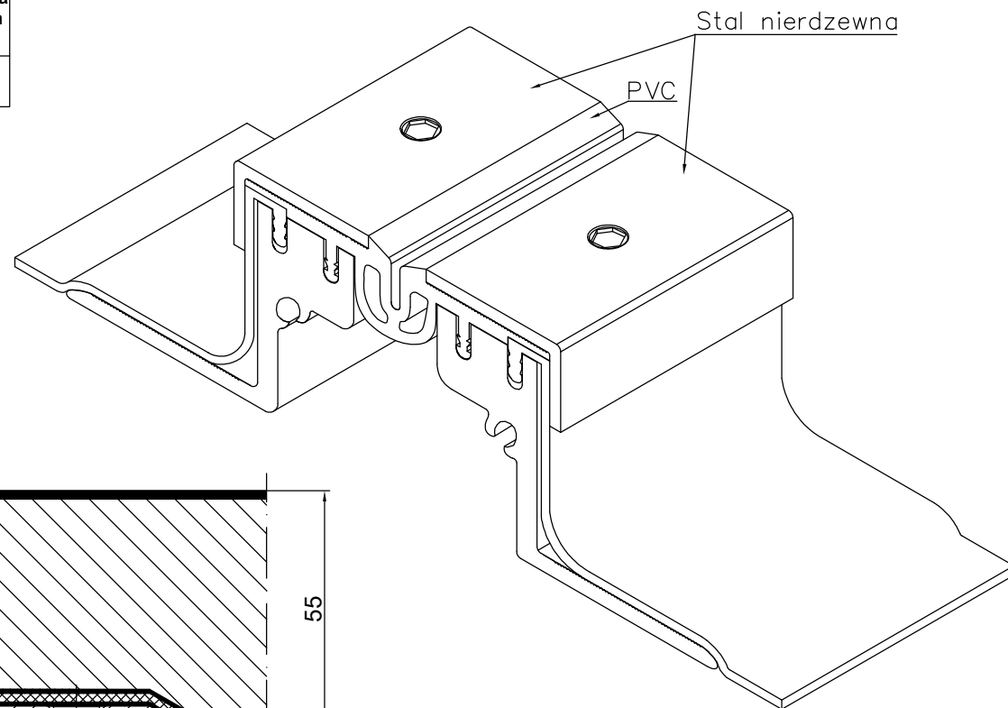
PROFIL DYLATACJNY GA 43.10.55 L RZUT AKSONOMETRYCZNY
