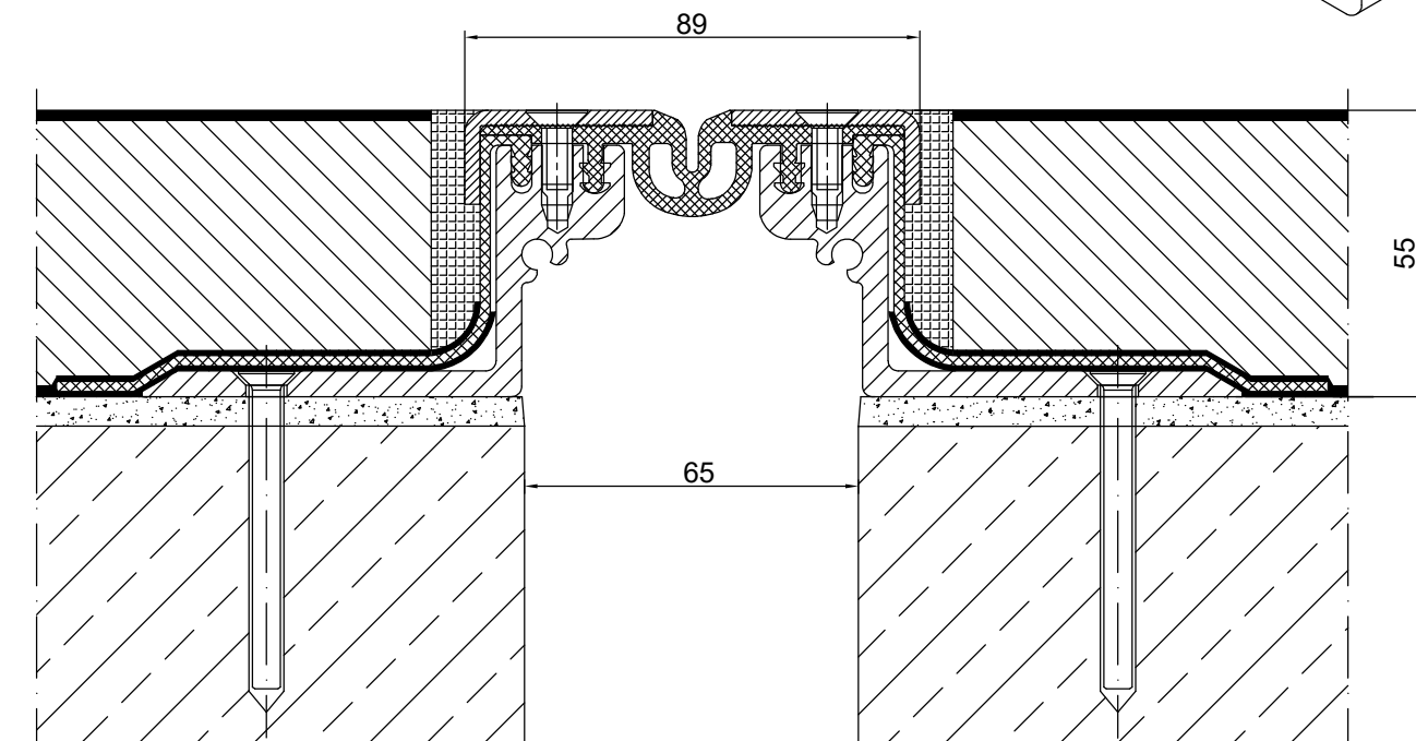
PROFIL DYLATACJNY GA 43.10.55 L PRZEKRÓJ
