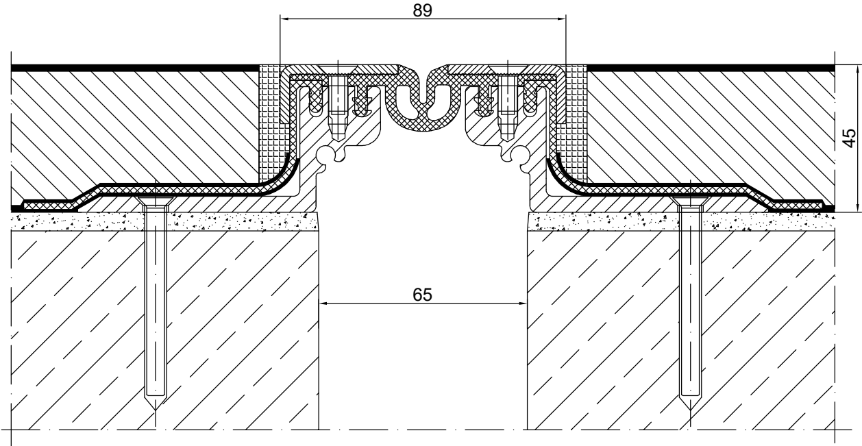
CONECTO GA 43.10.45 L PRZEKRÓJ
