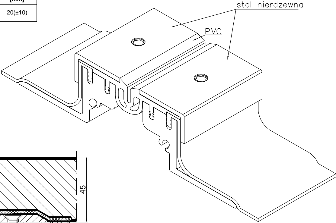
CONECTO GA 43.10.45 L RZUT AKSONOMETRYCZNY
