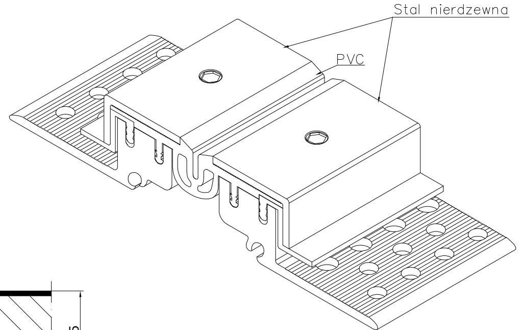
PROFIL DYLATACJNY GA 43.10.35 S RZUT AKSONOMETRYCZNY
