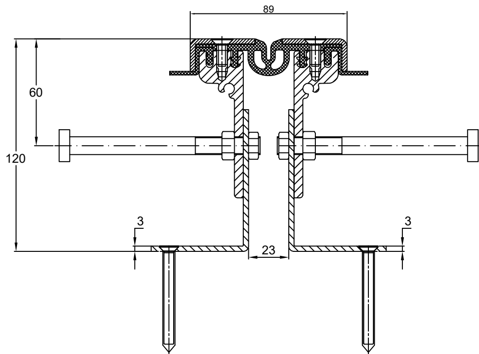
CONECTO PARK GA 43.10.120 S z ocynkowanymi ćwikami PRZĘKRÓJ
