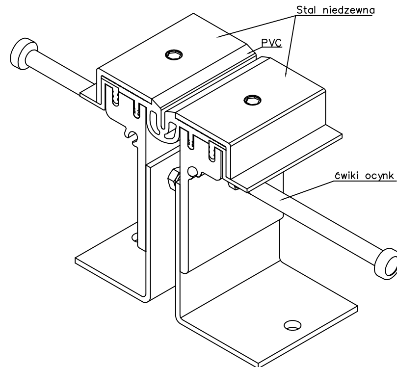
CONECTO PARK GA 43.10.120 S z ocynkowanymi ćwikami RZUT AKSONOMETRYCZNY
