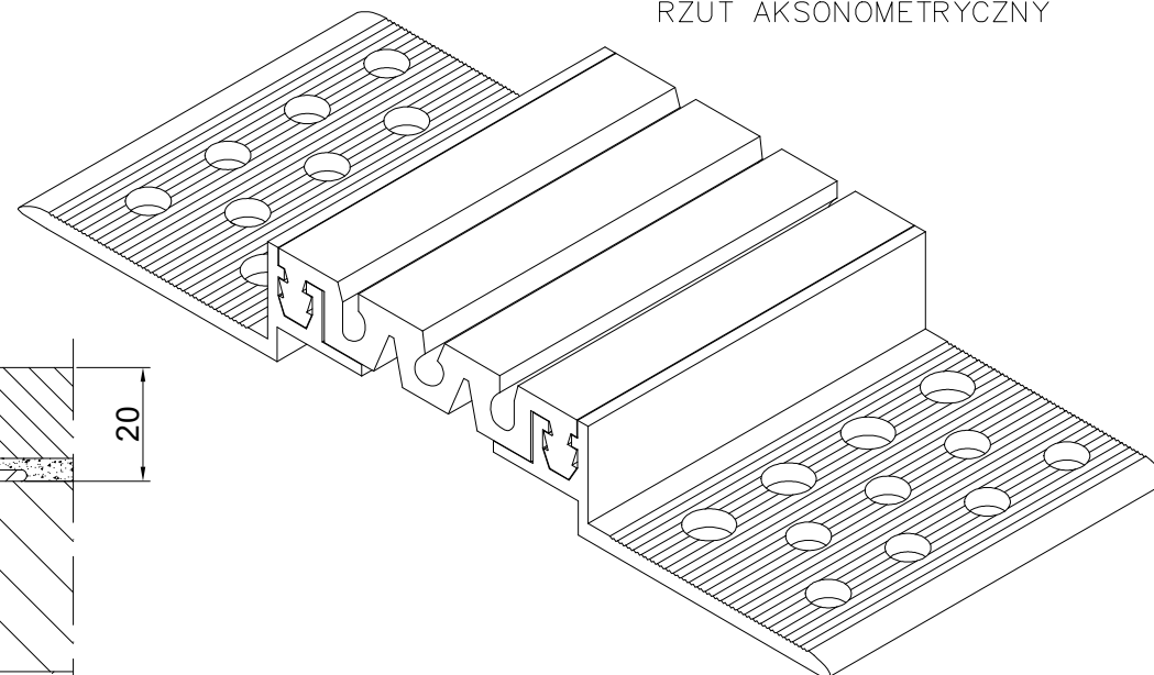
PROFIL DYLATACJNY EL 65.10.20 RZUT AKSONOMETRYCZNY
