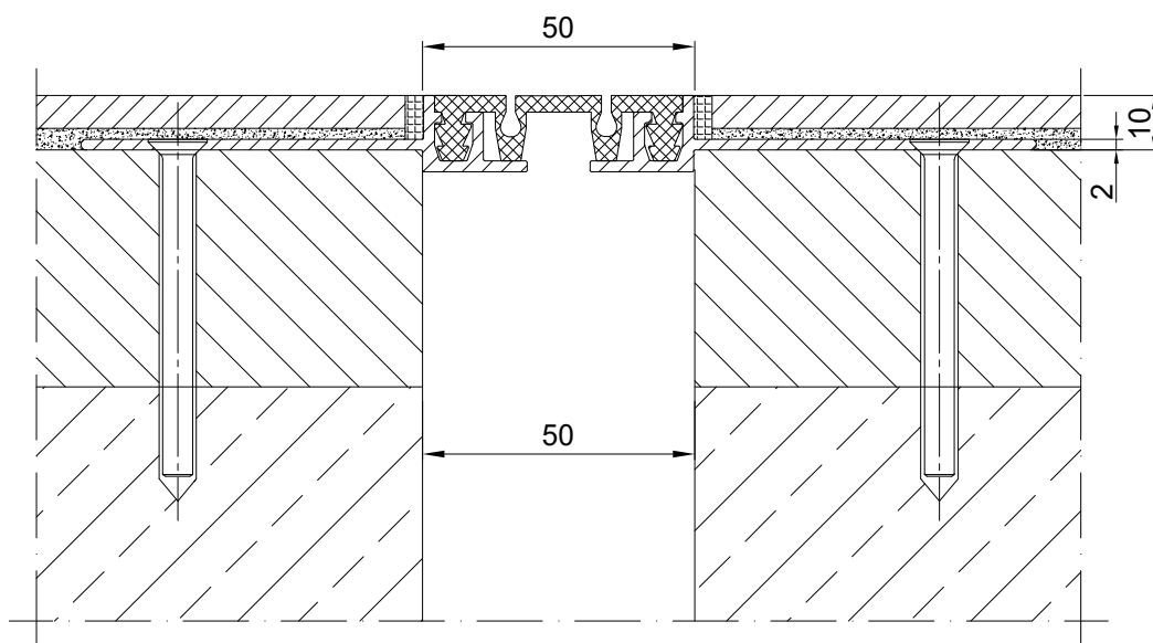
PROFIL DYLATACJNY EL 50.8.10 PRZEKRÓJ
