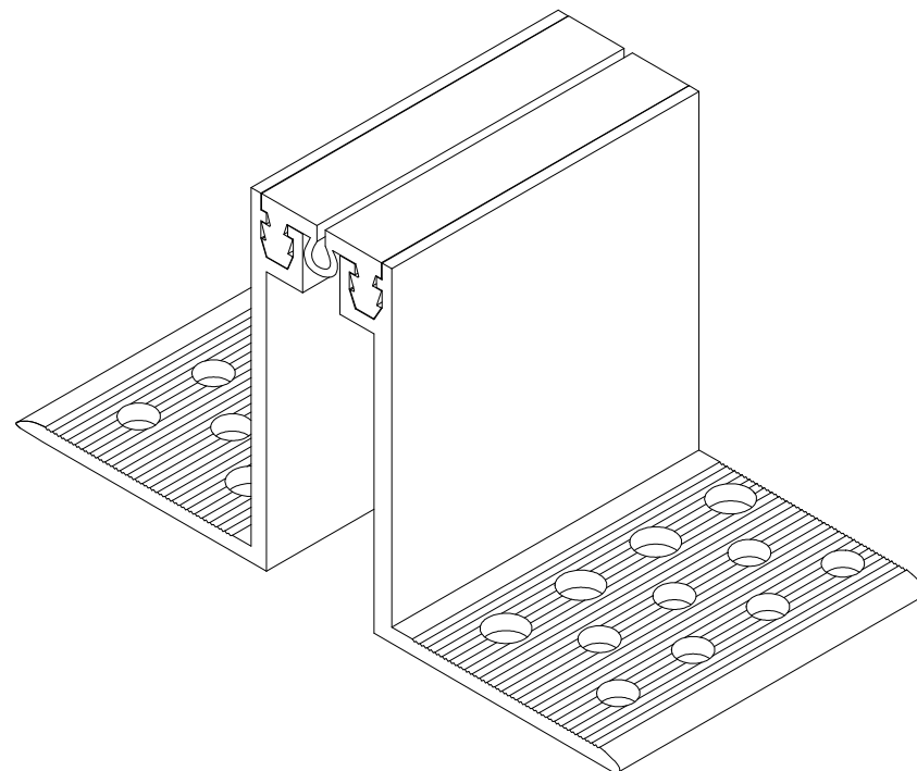
PROFIL DYLATACJNY EL 30.6.70 RZUT AKSONOMETRYCZNY
