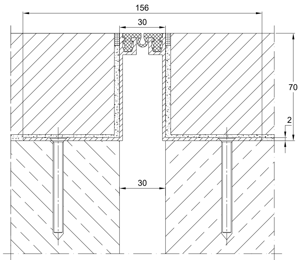
PROFIL DYLATACJNY EL 30.6.70 PRZEKRÓJ
