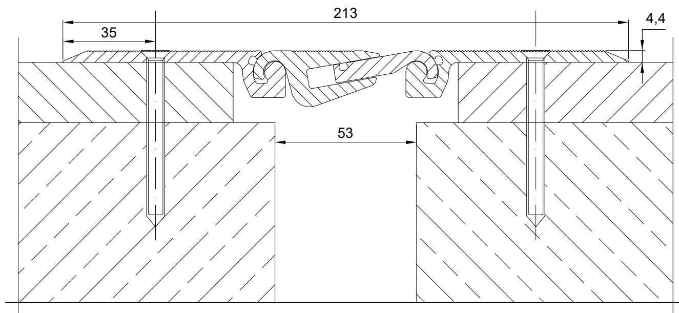
PROFIL DYLATACJNY AL 78.10.N PRZEKRÓJ
