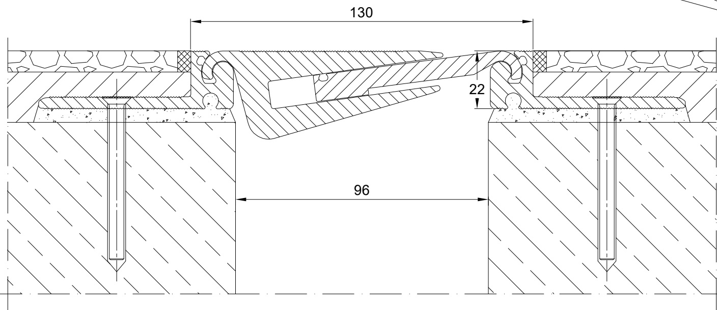
PROFIL DYLATACJNY AL 130.21.22 PRZEKRÓJ
