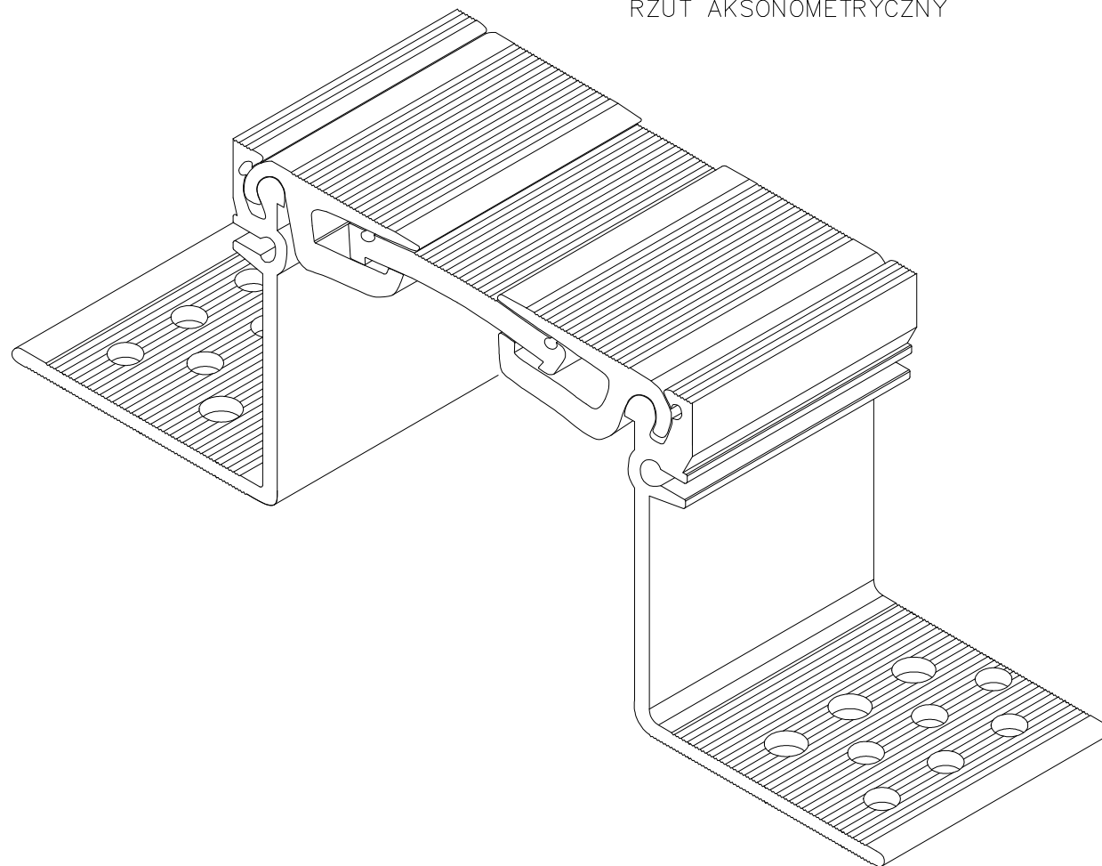
PROFIL DYLATACJNY AL 125.20.87 RZUT AKSONOMETRYCZNY
